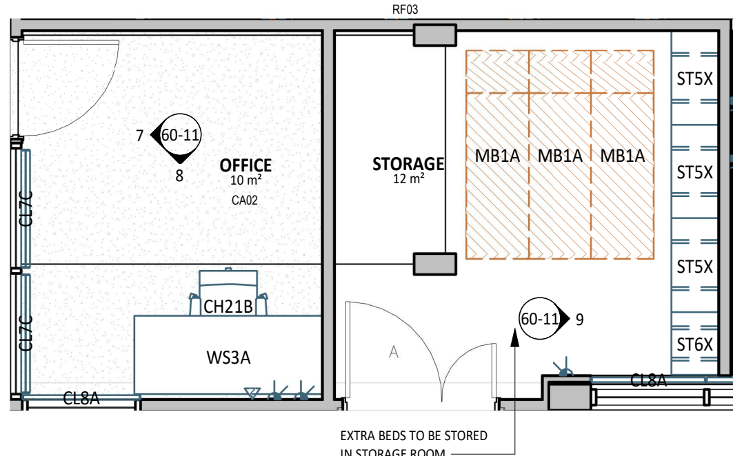
6 PLAN DETAIL 1 : 50
