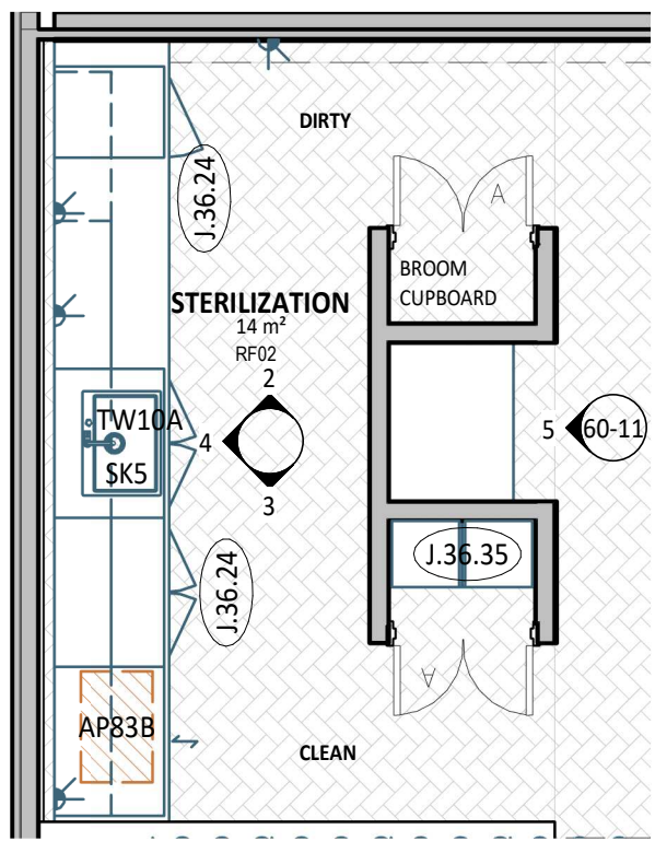
1 PLAN DETAIL 1 : 50
